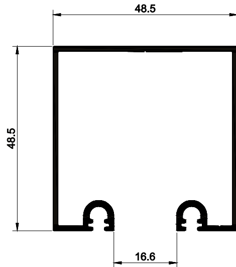
EVT-152 0,087 kg/m
