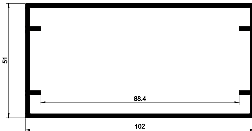
EPO-078L 0,654 kg/m
