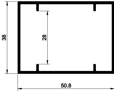
EPO-079 0,484 kg/m
