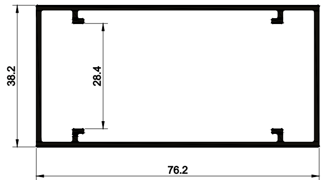
EPO-078 0,754 kg/m
