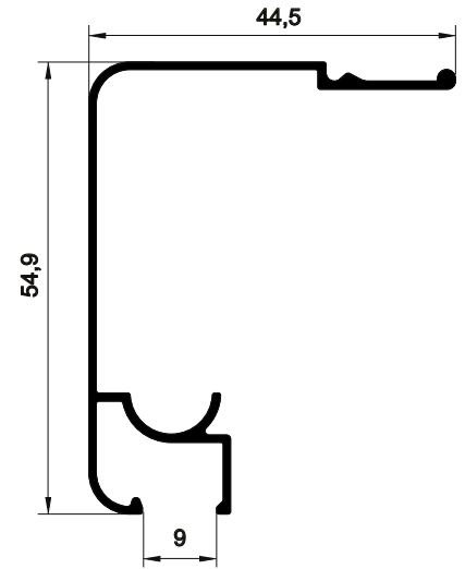
EVT-019 0,362 kg/m
