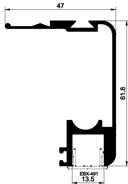
EVT-007 0,895 kg/m
