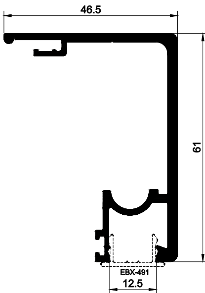
EVT-035 0,967 kg/m
