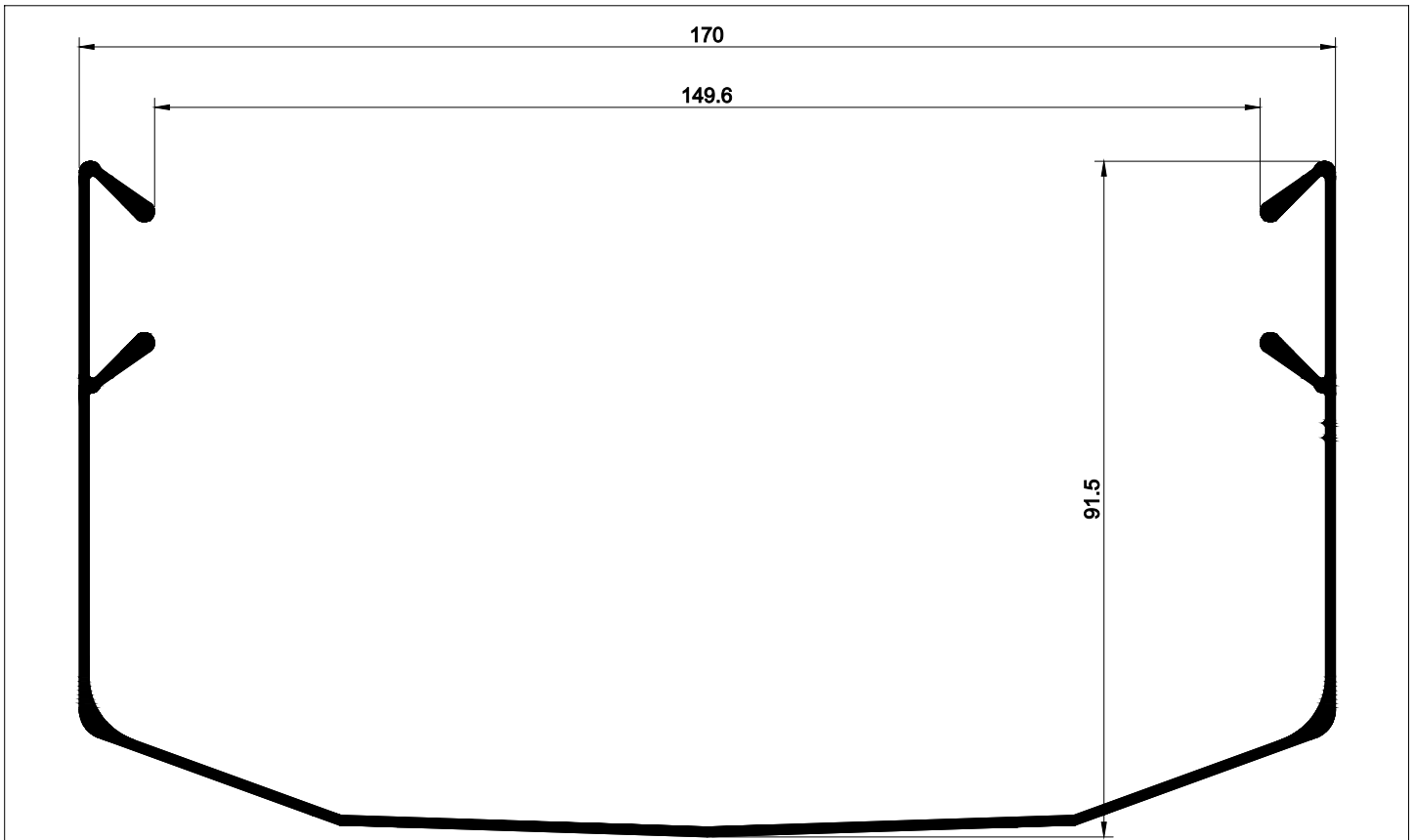
EDS-303 1,467 kg/m
