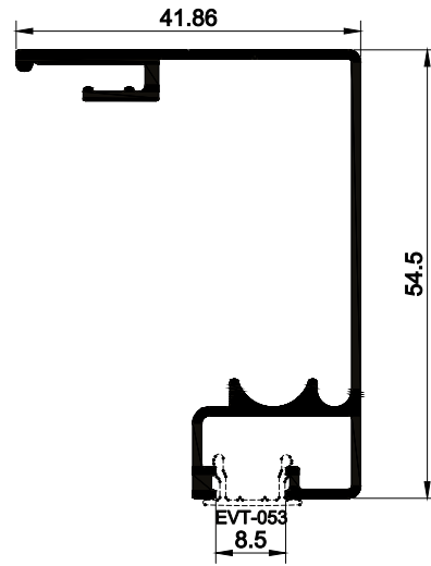
EVT-024 0,537 kg/m
