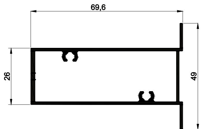
E90-586 0,577 kg/m
