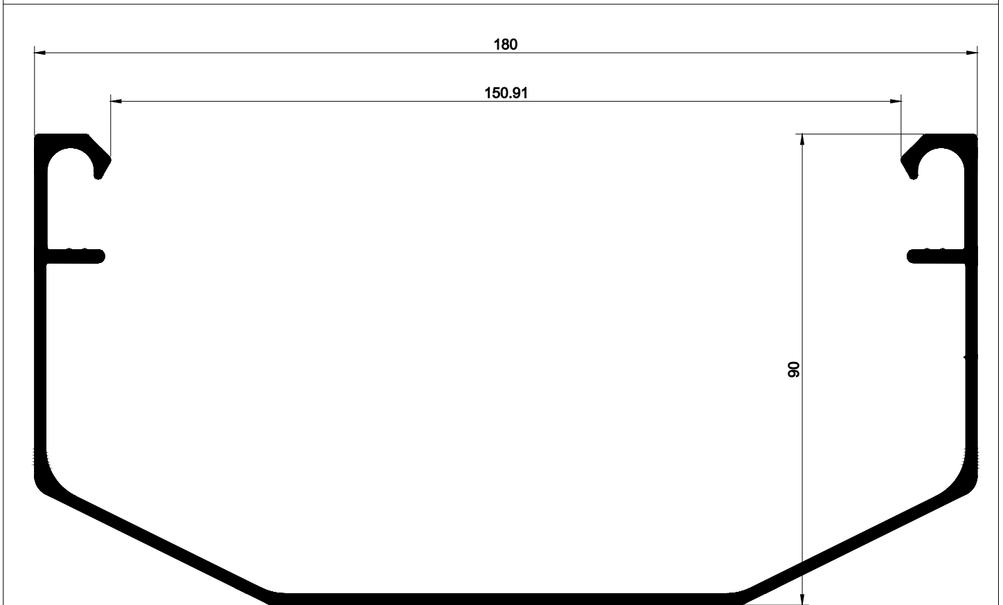
EDS-303 1,467 kg/m
