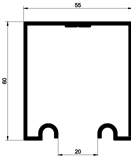
EVT-280 0,510 kg/m
