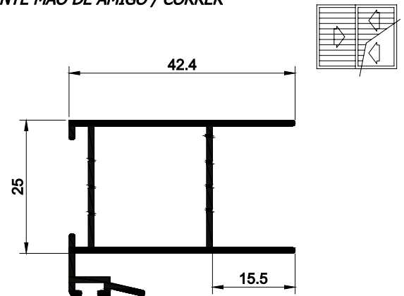
MONTANTE MÃO DE AMIGO / CORRER
