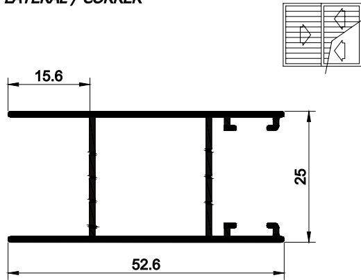
MONTANTE LATERAL / CORRER
