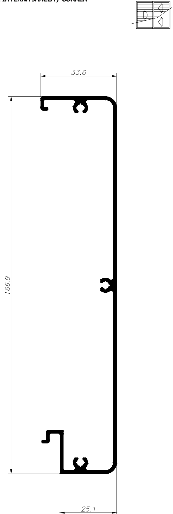
TAMPA INTERNA JANELA / CORRER
