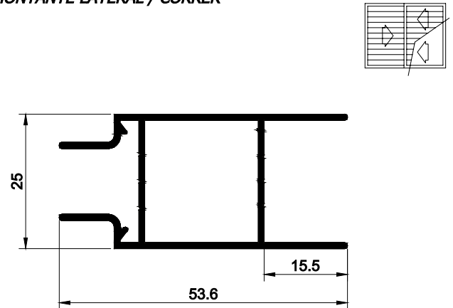
MONTANTE LATERAL / CORRER
