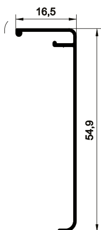
EVT-020 0,178 kg/m
