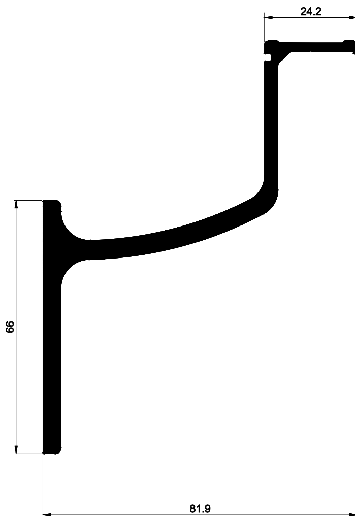
BASE CORRIMÃO
