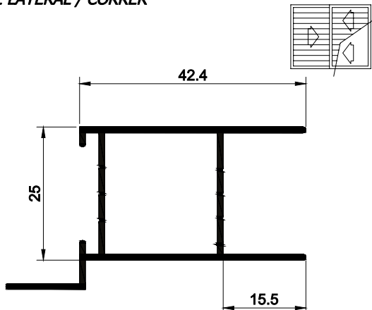
MONTANTE LATERAL / CORRER
