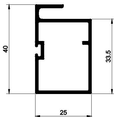
PERFIL TELA MOSQUITEIRA
