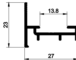
PERFIL MATA JUNTA / GIRO
