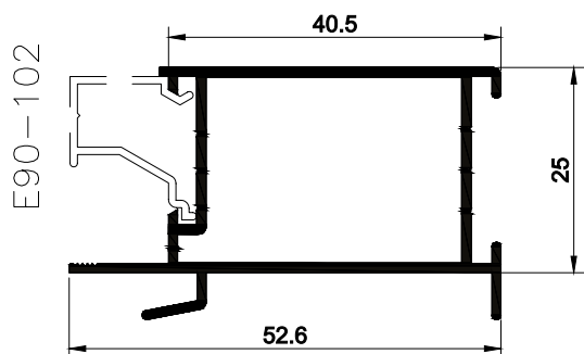
MONTANTE MÃO DE AMIGO / CORRER
