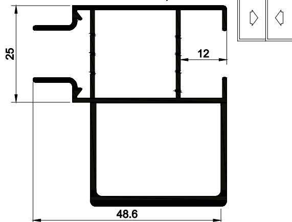
MONTANTE LATERAL SEM BAGUETE / CORRER
