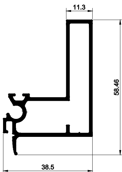
EFA-256 0,805 kg/m
