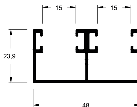
EVT-028 0,515 kg/m
