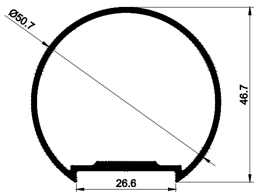
CORRIMÃO
