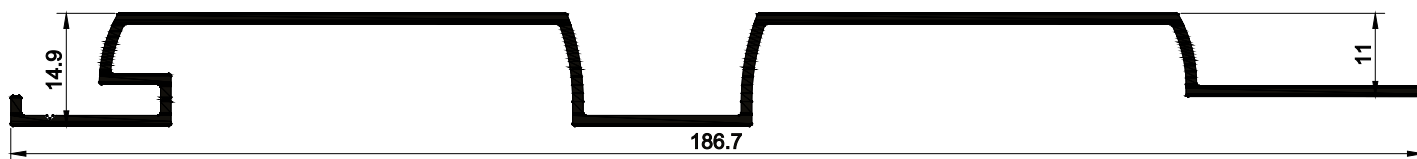
ELB-043 0,691 kg/m
