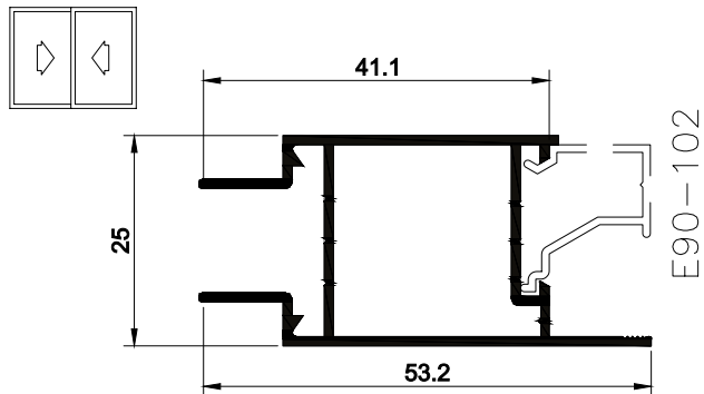
MONTANTE LATERAL FEC CENTRAL / CORRER
