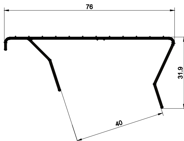
ESC-021 0,417 kg/m
