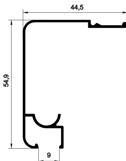
EVT-019 0,362 kg/m
