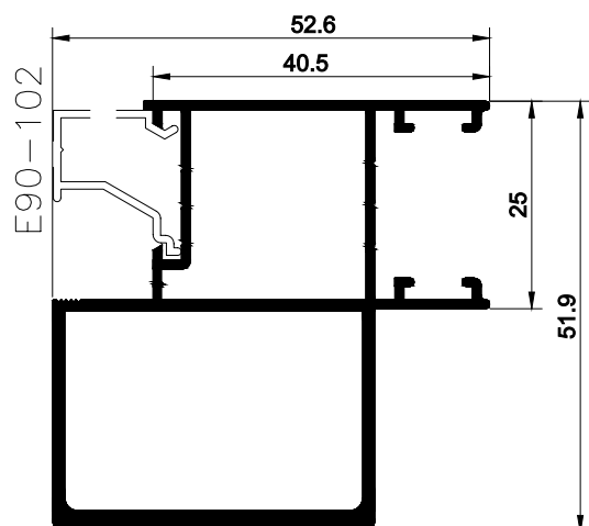
MONTANTE LATERAL COM REFORÇO / CORRER
