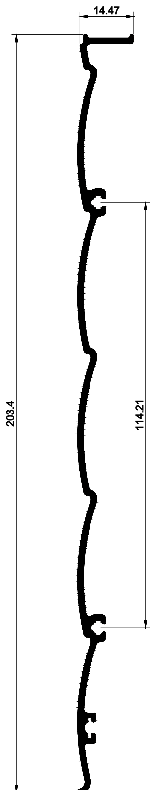
TAMPA EXTERNA PORTA / INTEGRADA
