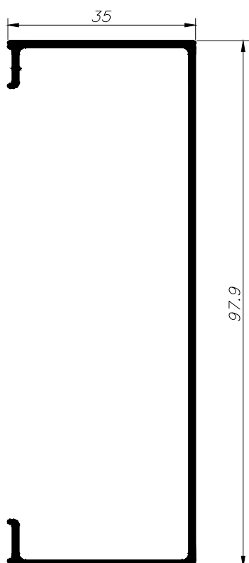
CAIXA FITA / CORRER
