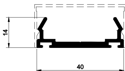
TAMPA PARA ARREMATE 42mm
