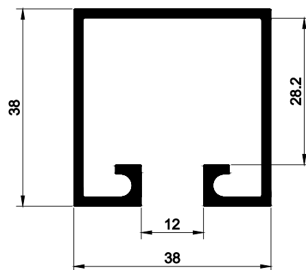
EPO-990 0,751 kg/m
