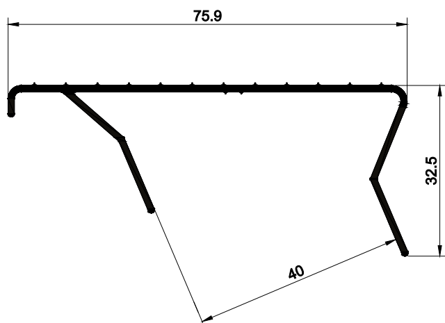
ESC-020 0,465 kg/m
