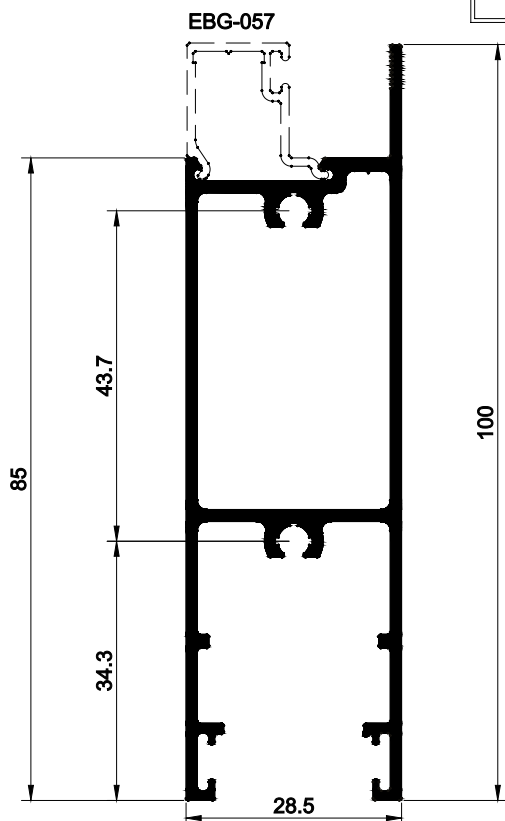
TRAVESSA INFERIOR / CORRER
