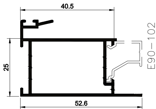
MONTANTE MÃO DE AMIGO / CORRER
