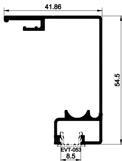
EBX-024 0,537 kg/m
