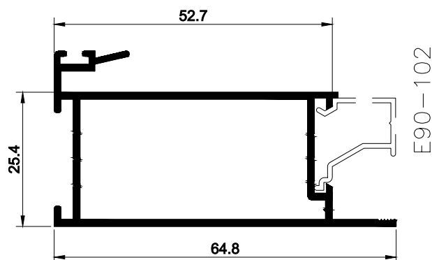
MONTANTE MÃO DE AMIGO / CORRER
