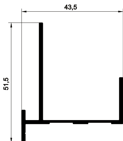
EIR-019 0,528 kg/m
