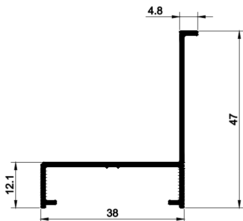
CONTRA MARCO
