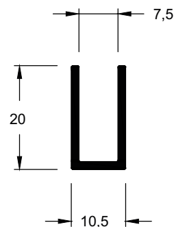
EPU-008 0,192 kg/m
