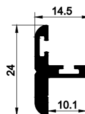
EPU-559 0,127 kg/m
