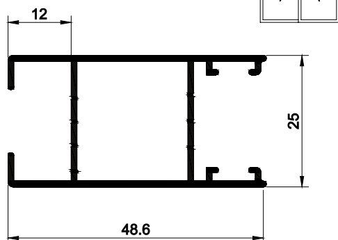
MONTANTE LATERAL SEM BAGUETE / CORRER
