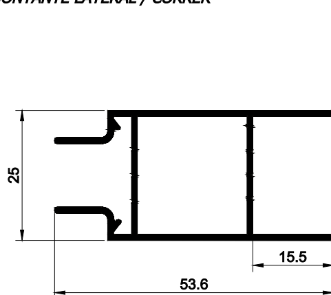
MONTANTE LATERAL / CORRER
