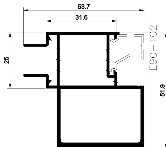
MONTANTE LATERAL / CORRER
