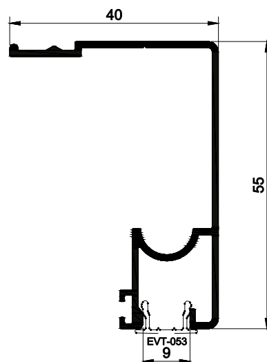
EVT-008 0,483 kg/m
