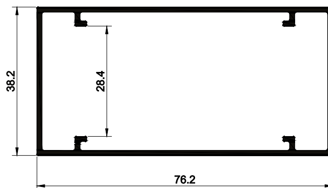
EPO-078 0,754 kg/m
