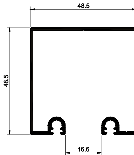
EVT-152 0,087 kg/m
