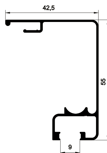
EVT-081 0,473 kg/m
