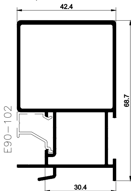
MONTANTE MÃO DE AMIGO REF / CORRER
